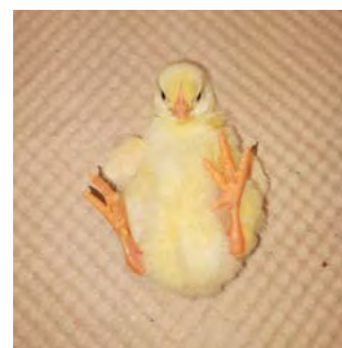
图4：活跃性
